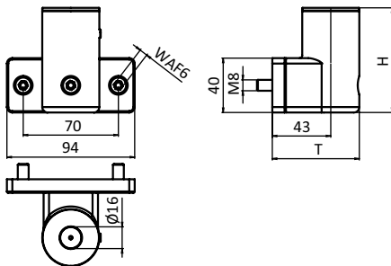
Side Adapter for Magnifying Lamp D160 with Jointed Arm (Set) Seiten-Adapter für Lupenleuchte D160 mit Gelenkarm (Set)
