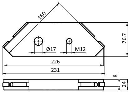
Bracing Plate 90° Stabilisierungsplatte 90°
