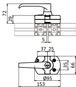
Türschloss (Set) Door Lock (Set)
