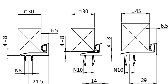
Dichtleiste Sealing Strip
