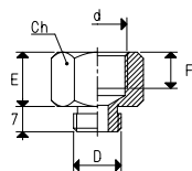
RIDUZIONE MF PER VENTOSE VRP-VRS-VEP-VE MF REDUCTIONS FOR VRP-VRS-VEP-VE CUPS
