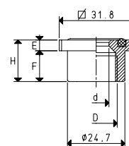
ADATTATORE QUADRO PER VENTOSE VRP-VRS-VEP-VE SQUARE ADAPTER FOR VRP-VRS-VEP-VE CUPS
