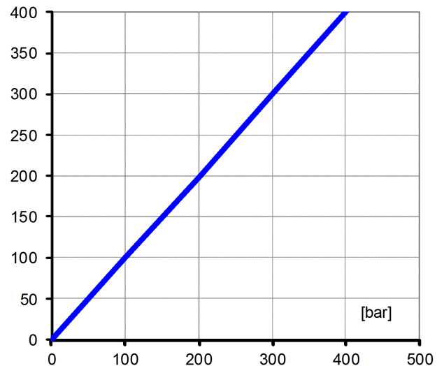
F[ N] Diagramma Pressione-Forza; L=300 Diagram Pressure-Force; L=300
