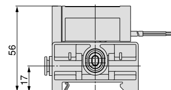
Blocco di alimentazione comune con pressostato (P)
