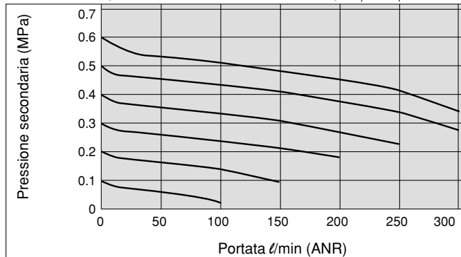
ARM11AA1-312 (Rac. istantanei: entrata ø10, uscita ø6) Condizioni: pressione primaria 0.7 MPa
