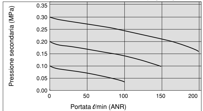
ARM11AA1-310-1 (Rac. istantanei: entrata ø8, uscita ø6) Condizioni: pressione primaria 0.5 MPa
