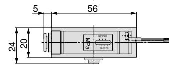
Blocco di alimentazione comune valvola 3 vie + Blocco pressostato (W)
