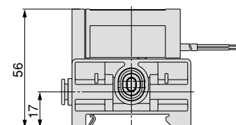
Blocco di alimentazione comune valvola 3 vie + Blocco pressostato (W)
