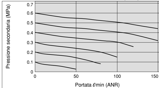
ARM11AA1-307 (Rac. istantanei: entrata ø6, uscita ø4) Condizioni: pressione primaria 0.7 MPa
