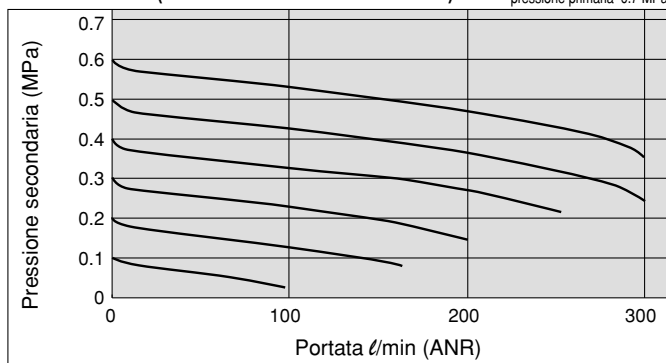
ARM11BA1-308 (Rac. istantanei: entrata/uscita ø6) Condizioni: pressione primaria 0.7 MPa
