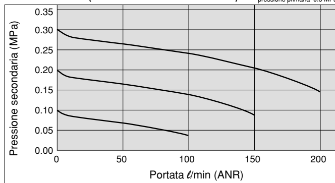
ARM11BA1-308-1 (Rac. istantanei: entrata/uscita ø6) Condizioni: pressione primaria 0.5 MPa
