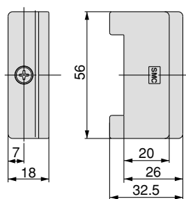
Blocco finale lato R
