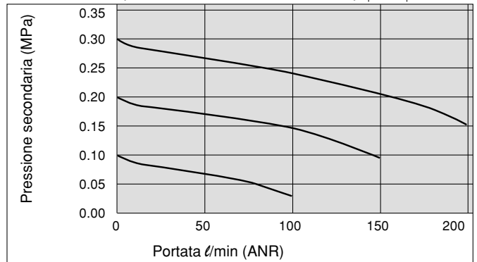
ARM11AA1-312-1 (Rac. istantanei: entrata ø10, uscita ø6) Condizioni: pressione primaria 0.5 MPa
