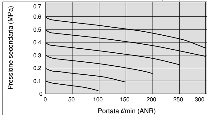
ARM11AA1-310 (Rac. istantanei: entrata ø8, uscita ø6) Condizioni: pressione primaria 0.7 MPa
