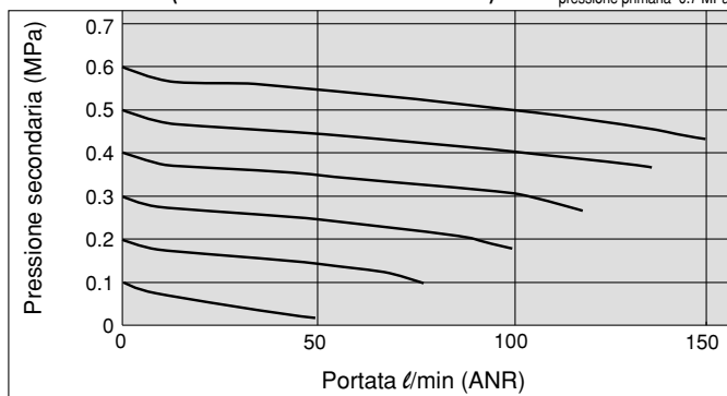
ARM11BA1-306 (Rac. istantanei: entrata/uscita ø4) Condizioni: pressione primaria 0.7 MPa
