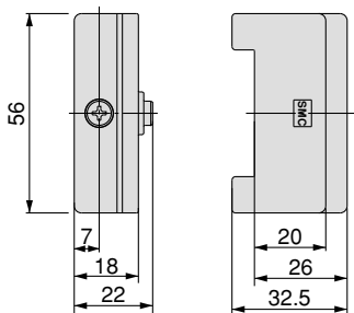
Blocco finale lato L
