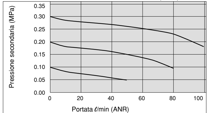
ARM11AA1-307-1 (Rac. istantanei: entrata ø6, uscita ø4) Condizioni: pressione primaria 0.5 MPa
