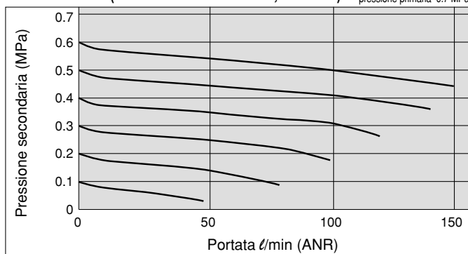
ARM11BA1-307 (Rac. istantanei: entrata ø6, uscita ø4) Condizioni: pressione primaria 0.7 MPa
