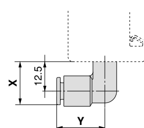
Modello a gomito
