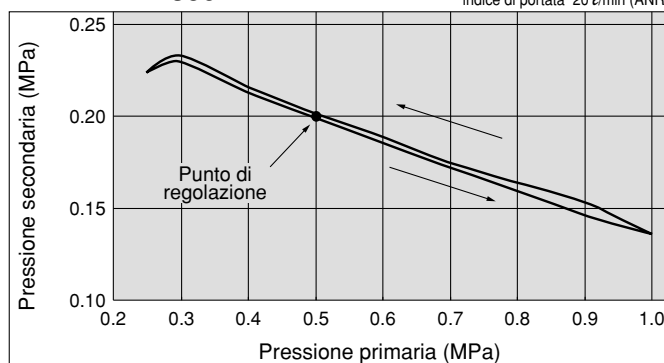
ARM11BA1-306-1 Condizioni: pressione primaria 0.5 MPa pressione secondaria 0.2 MPa indice di portata 20 l/min (ANR)
