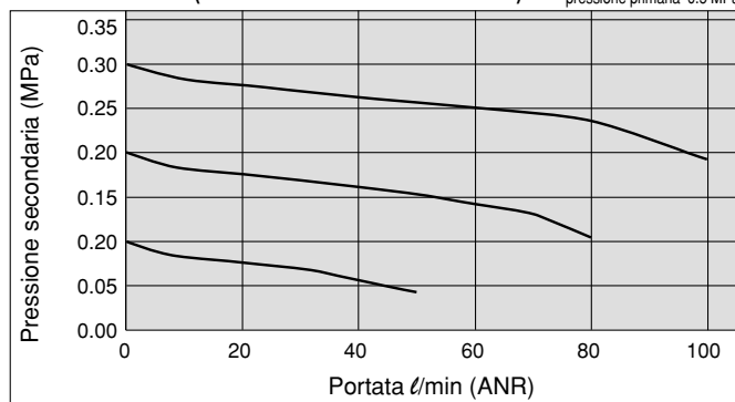
ARM11BA1-306-1 (Rac. istantanei: entrata/uscita ø4) Condizioni: pressione primaria 0.5 MPa
