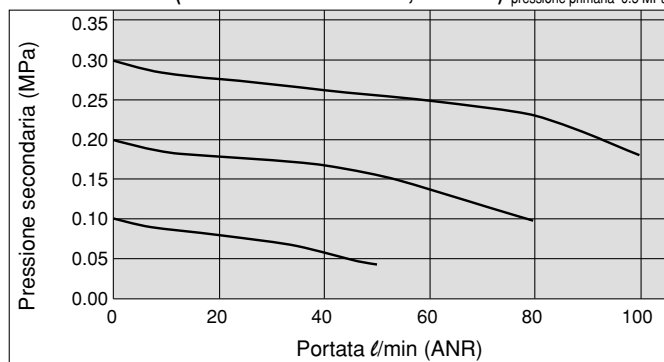
ARM11BA1-307-1 (Rac. istantanei: entrata ø6, uscita ø4) Condizioni: pressione primaria 0.5 MPa
