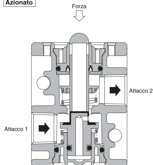
Azionato
