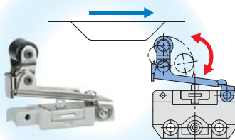
Leva a rullo unidirezionale
