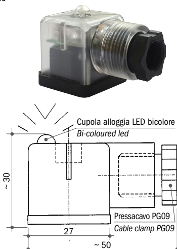
Connettore trasparente con Led bicolore rosso/verde Transparent connector with red/green bi-coloured led Tipo CLB Type
