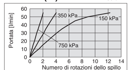
PF2M750(-L)
